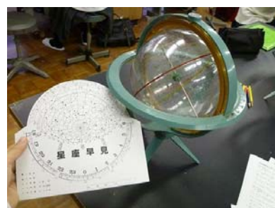
天球儀と手作りの星座早見盤
