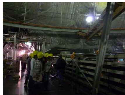
スーパーカミオカンデ内を見学
