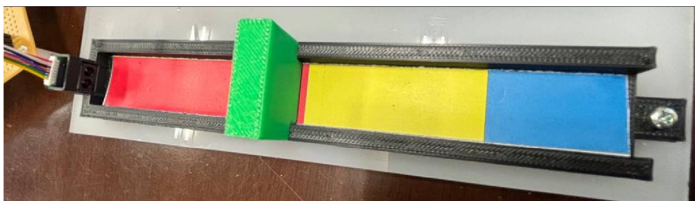
図7 測距用スライダ装置、 スライダー、 測距センサ設置図
